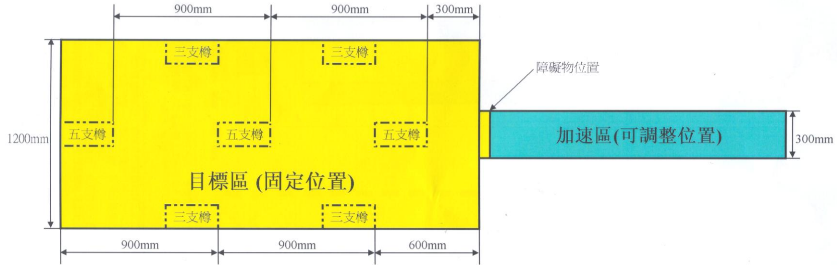
場區平面圖
